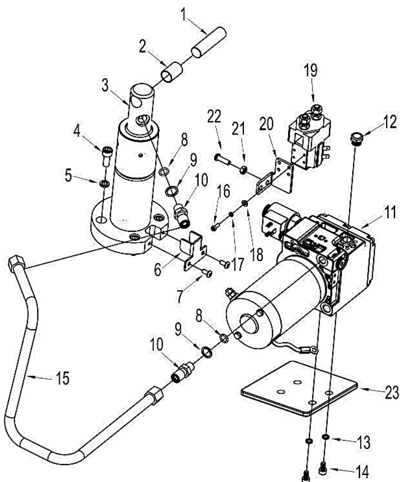
Схема 5. Гидравлика в сборе.
