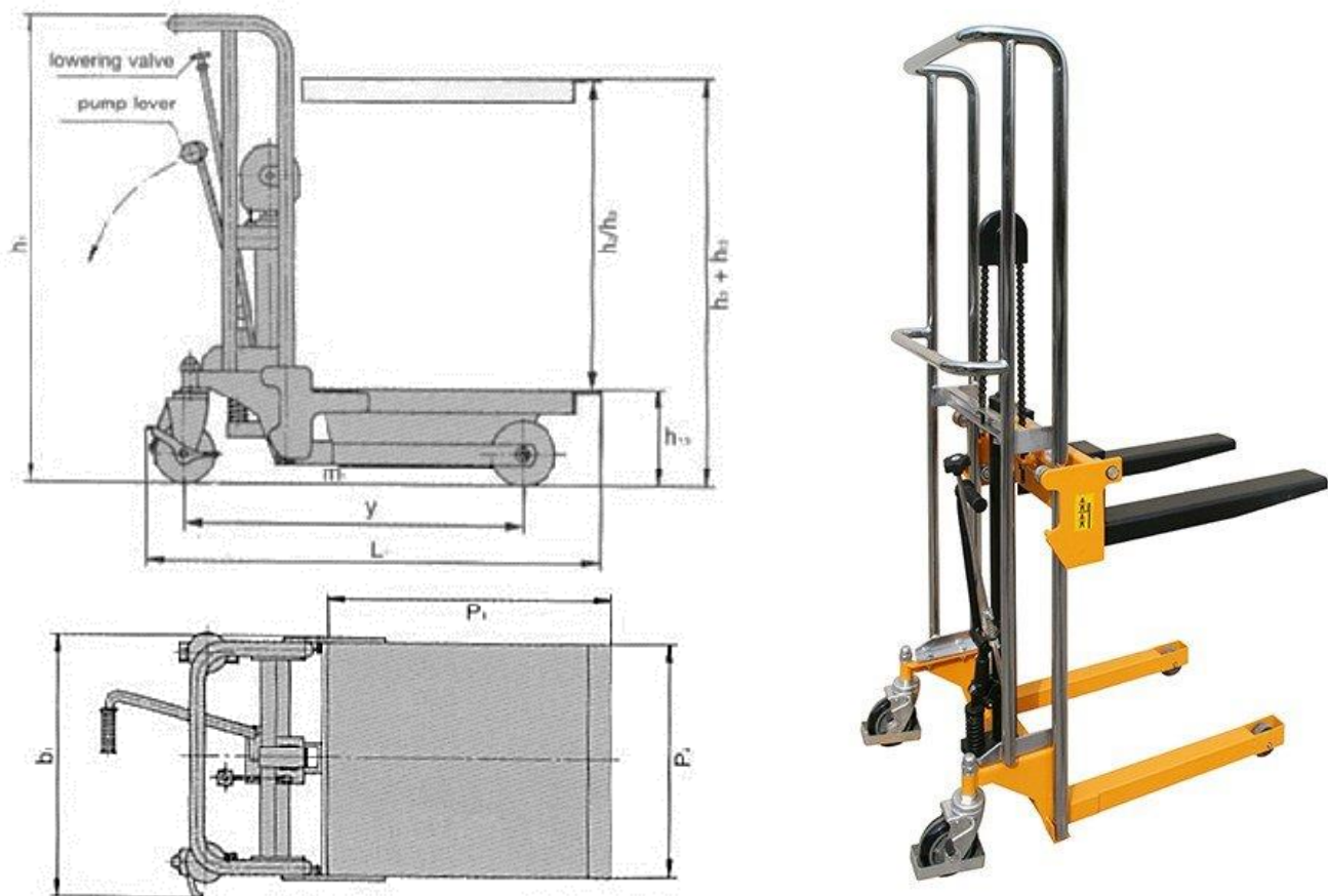
Рисунок 2. Габаритные размеры штабелера ручной PJ4150.
